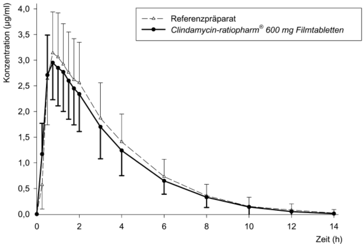
Abb.: Mittelwerte und Standardabweichungen der Plasmakonzentration von Clindamycin nach Einmalgabe von 1 Filmtablette Clindamycin-ratiopharm® 600 mg Filmtabletten bzw. 2 Kapseln Referenzpräparat mit jeweils 300 mg Clindamycin (entsprechend 600 mg Clindamycin).
