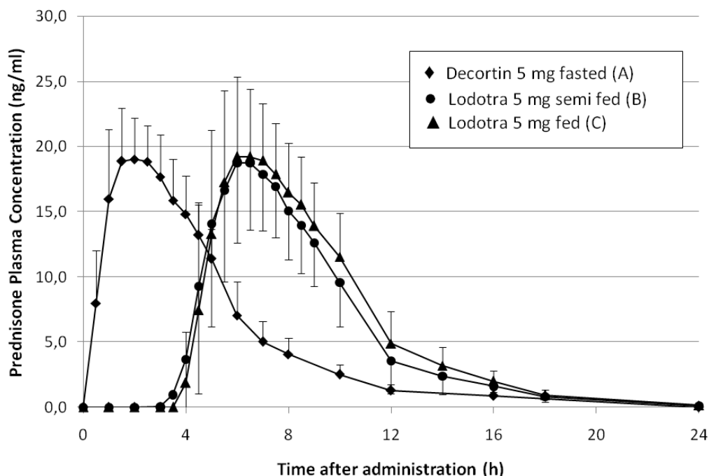
Abbildung: Mittlere Prednison-Plasmaspiegel nach einer Einzeldosis von 5 mg Prednison, verabreicht als Lodotra 5 mg oder als Tabletten mit sofortiger Wirkstofffreisetzung:
