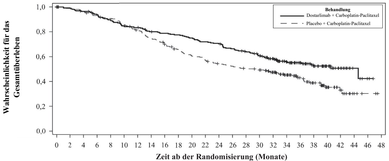
Abbildung 2: Kaplan-Meier Kurve des Gesamtüberlebens bei allen Patientinnen (Gesamtpopulation) mit EC (RUBY-Studie)
