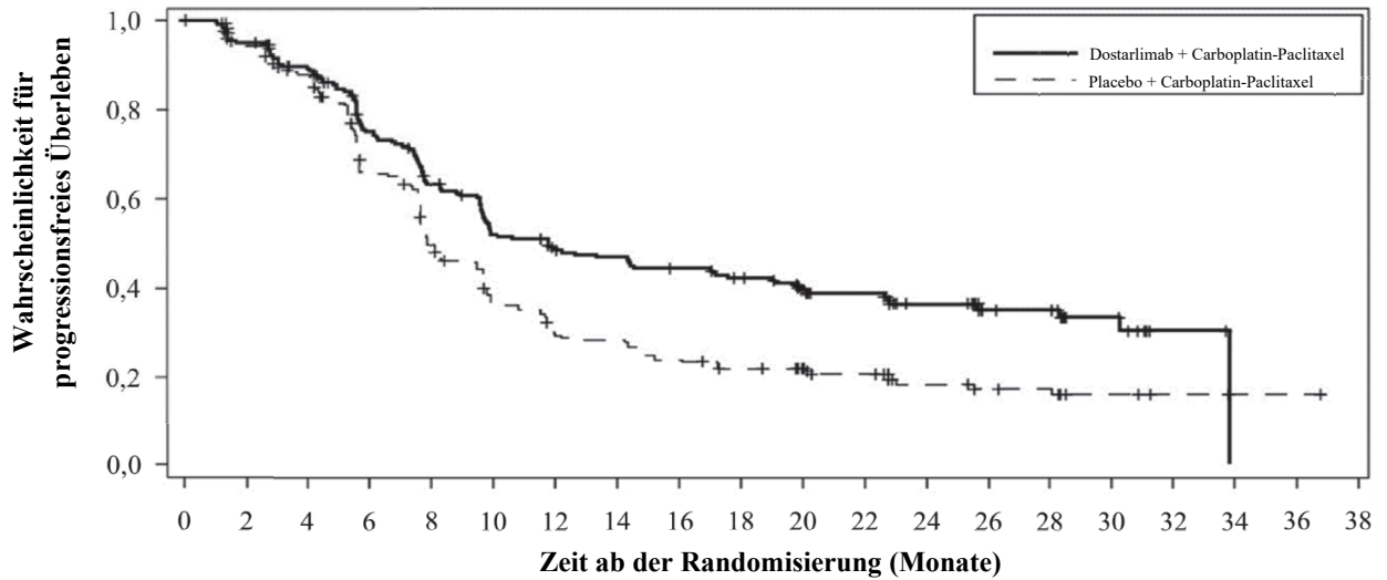
Anzahl der gefährdeten Personen (Anzahl an Ereignissen)
