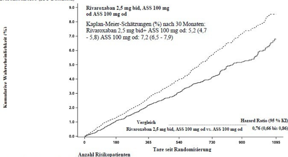
Kaplan-Meier-Darstellung der kumulativen Rate des primären Wirksamkeitsendpunktes bis zum Stichtag aller Ergebnisse zu Rivaroxaban/ASS (ITT-Datensatz)
